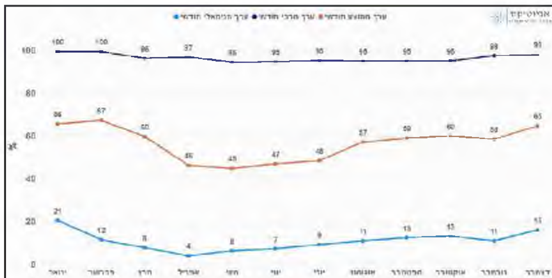
איור 4- שכיחות לחות חודשית שנמדדה בתחנת ירושלים, מרכז בין ה 1 לינואר 2021 עד 31 לדצמבר 2025
