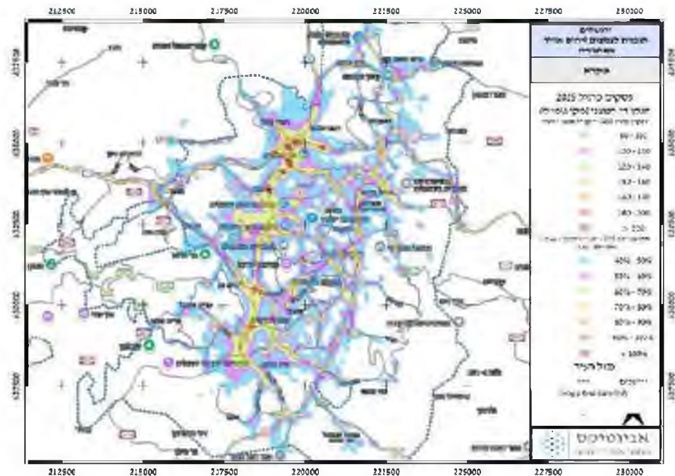
איור 14 - ריכוזים שחתיים מרביים צפויים לחקוק דו חמצני בירושלים לשנת 2025
