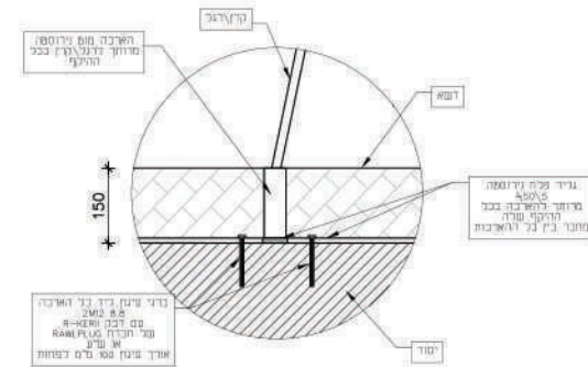
פרס עיגון קרניים קנ"מ 1:10 מידות במ"מ
