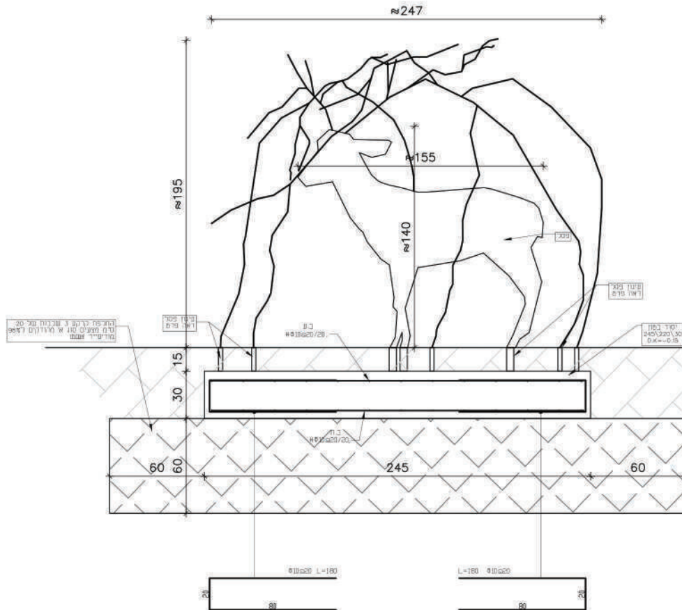
חתך 1-1 קנ"מ 1:20
