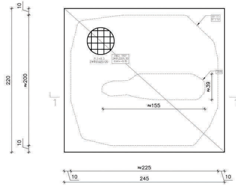
תכנית קנ"מ 1:20
